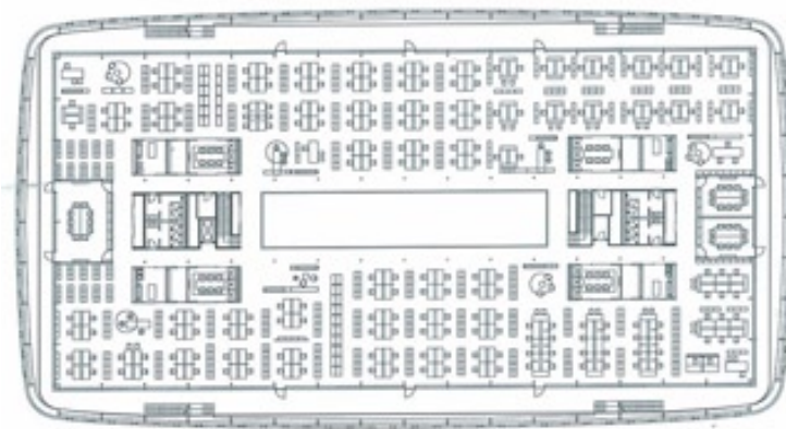
Grundriss 1. Obergeschoss First floor plan
